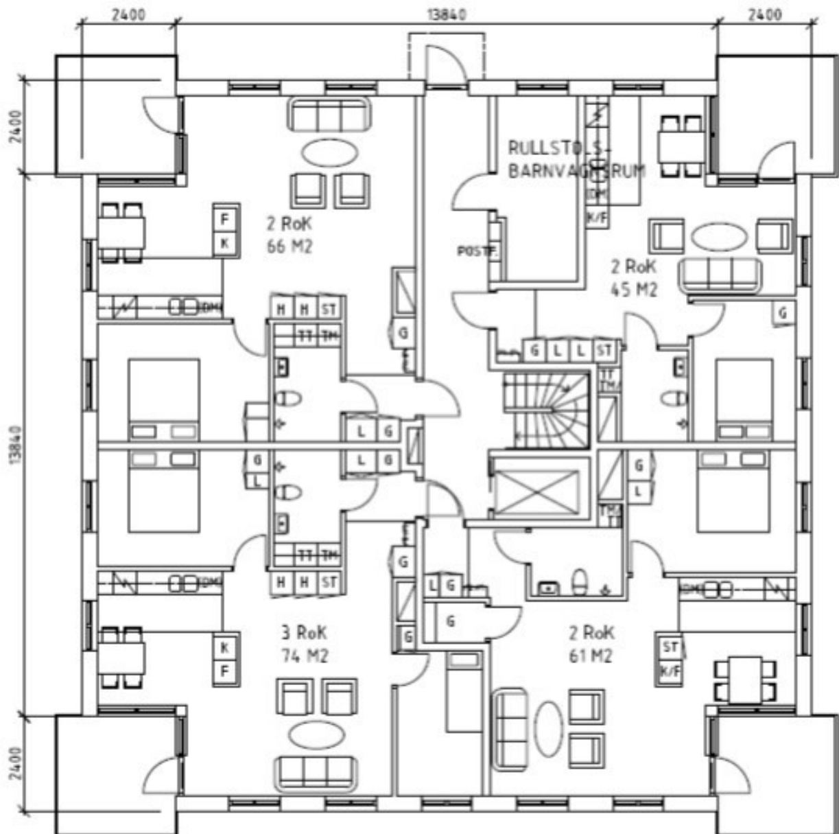
BOTTENVÅNING PLAN 1
