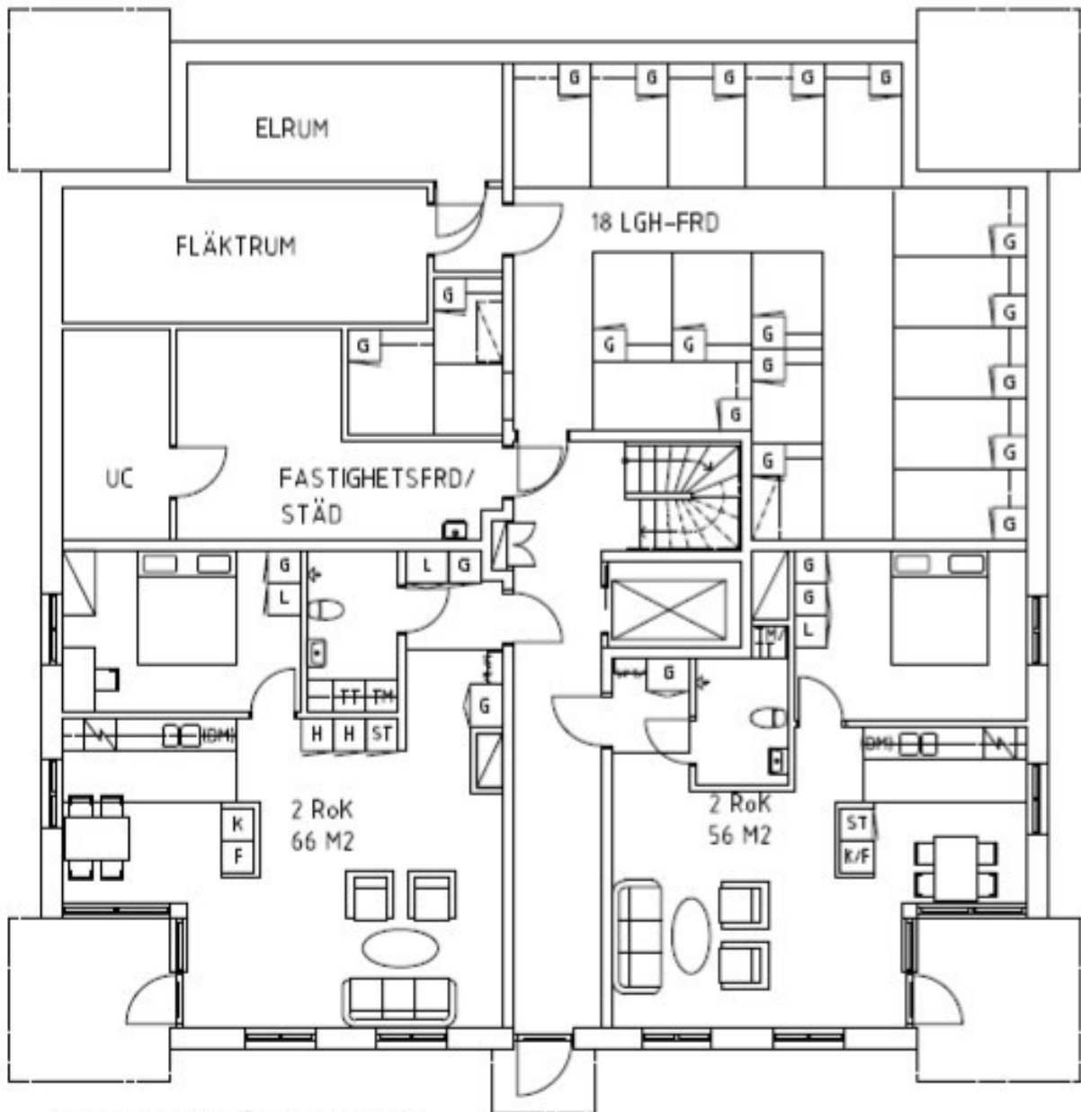
SUTTERÄNGVÅNING PLAN 0
